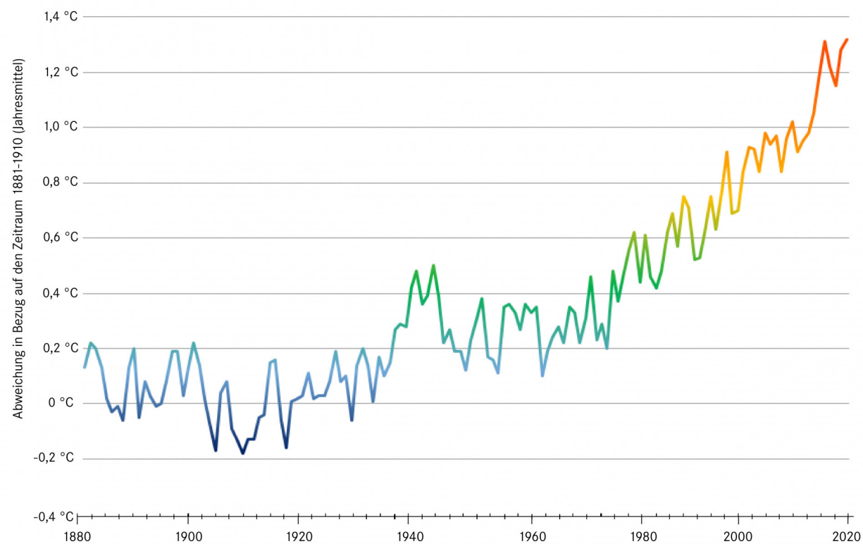
GLOBALE MITTELTEMPERATUR 1880-2020
