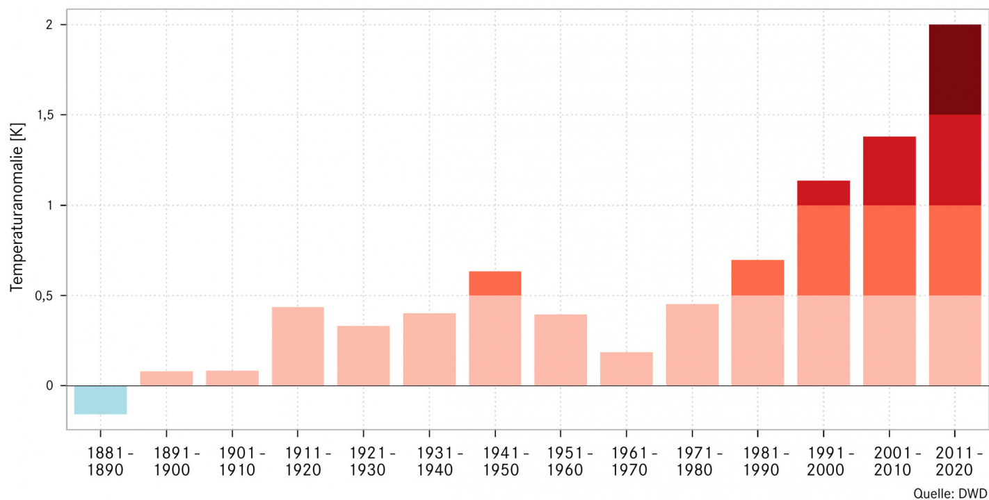
TEMPERATURANOMALIE DER 10-JAHRESPERIODEN DEUTSCHLAND REFERENZZEITRAUM 1881 - 1910
